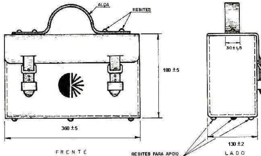
Desenho orientativo – Dimensões em milímetros
